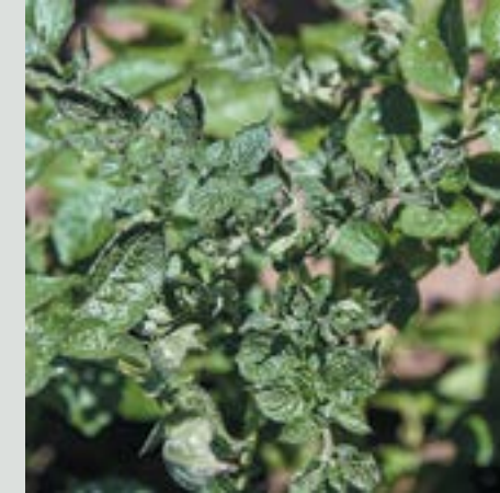
2, 4-D
