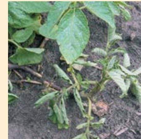
Flumioxazin
